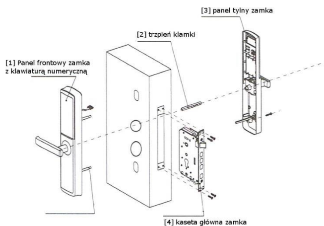
Rysunek 3. Montaż
