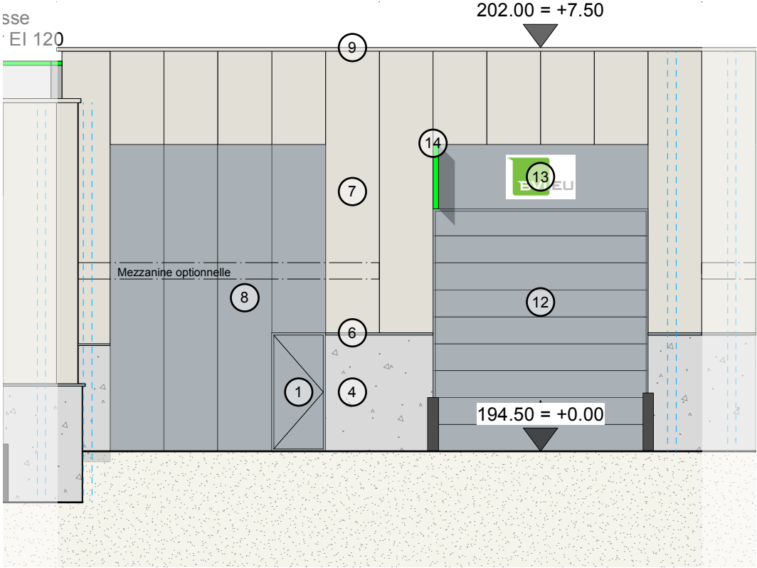
Elévation OUEST : 1/ 100
