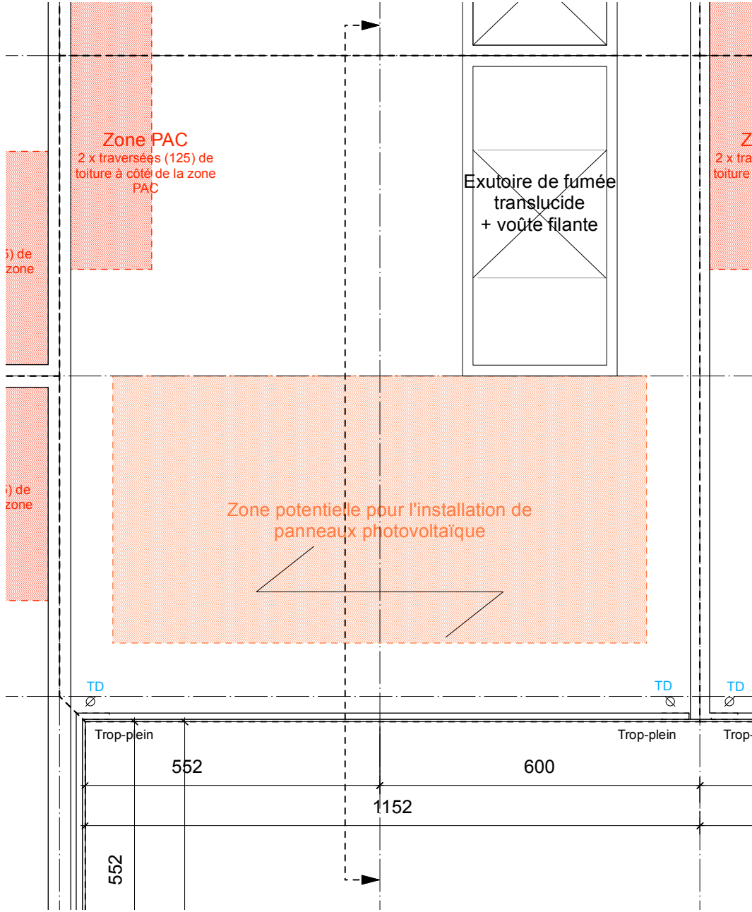
Plan de toiture : 1/ 100
