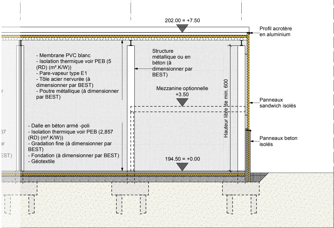
Coupe : 1/ 100
