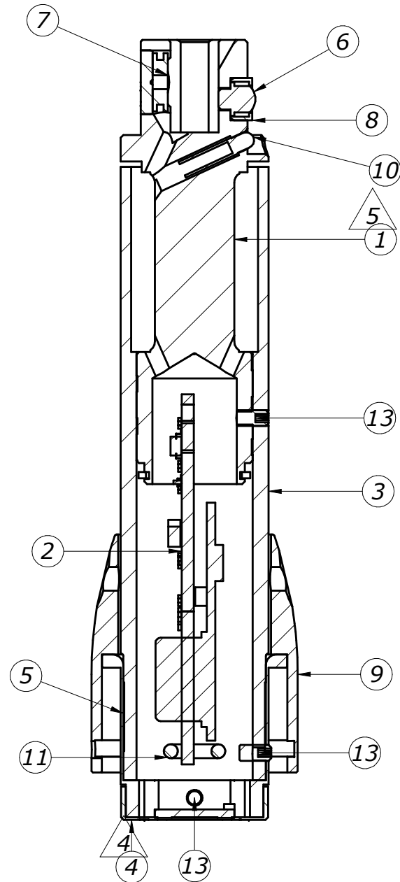
SEZIONE A-A
