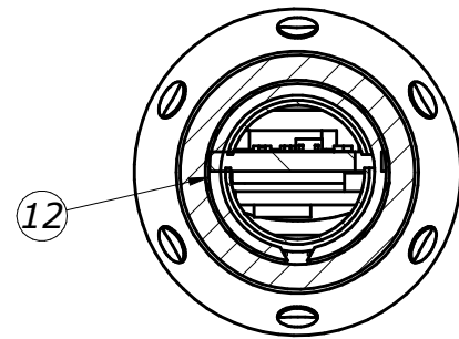
SEZIONE B-B
