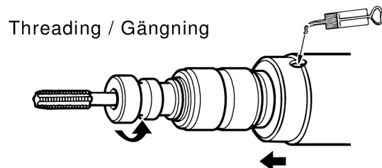
Threading / Gängning
