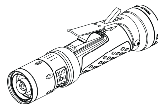
Fig. 2: Position déverrouillée.
