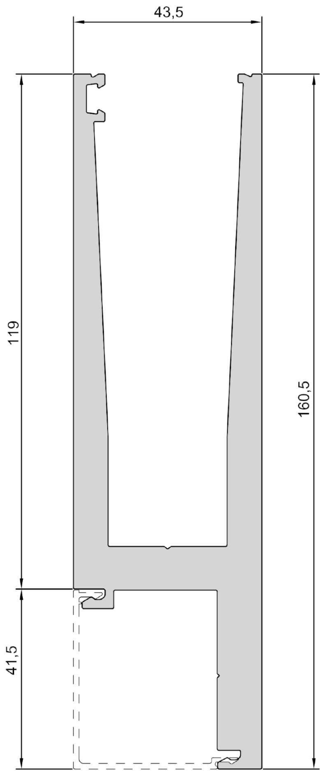
Y-PROFIL 1049
