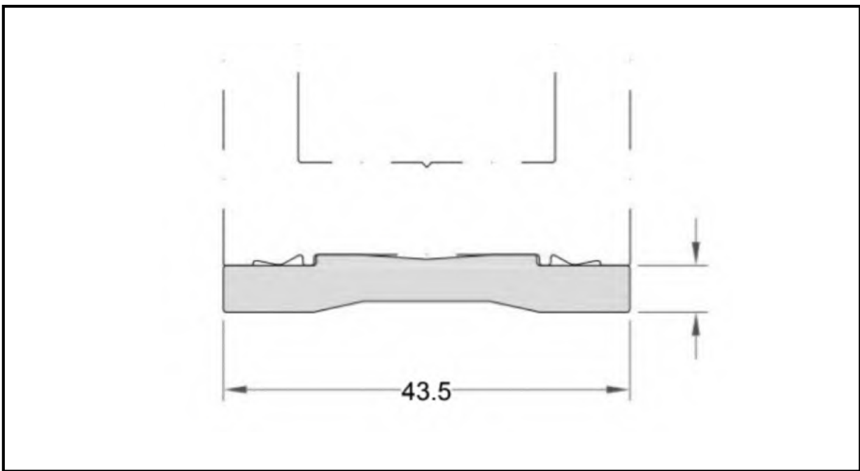
DRENERINGSPROFIL 1048
