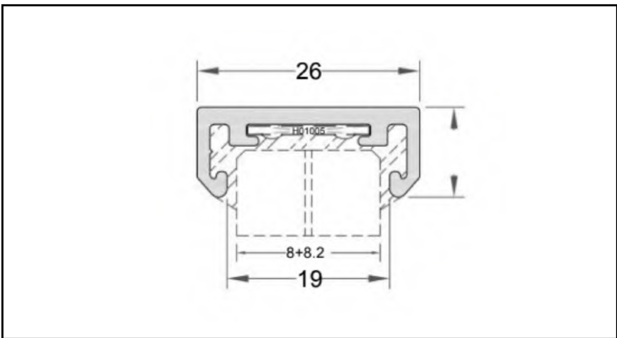
HÅNDLØPER 1054
