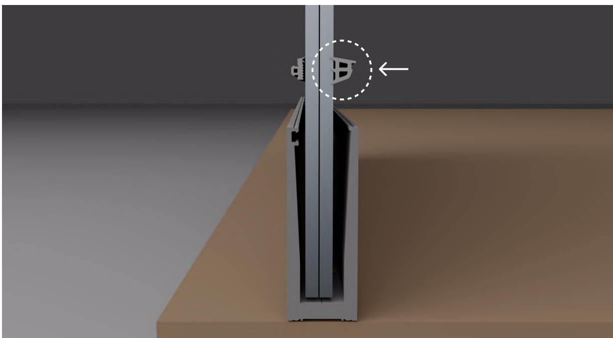
GUMMIPAKNING INNVENDIG (H08050)
