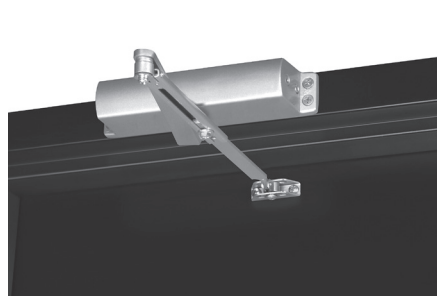
Top Jamb
