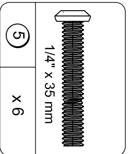
BOLT TCS1060
