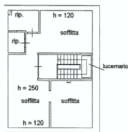
Piano Secondo
