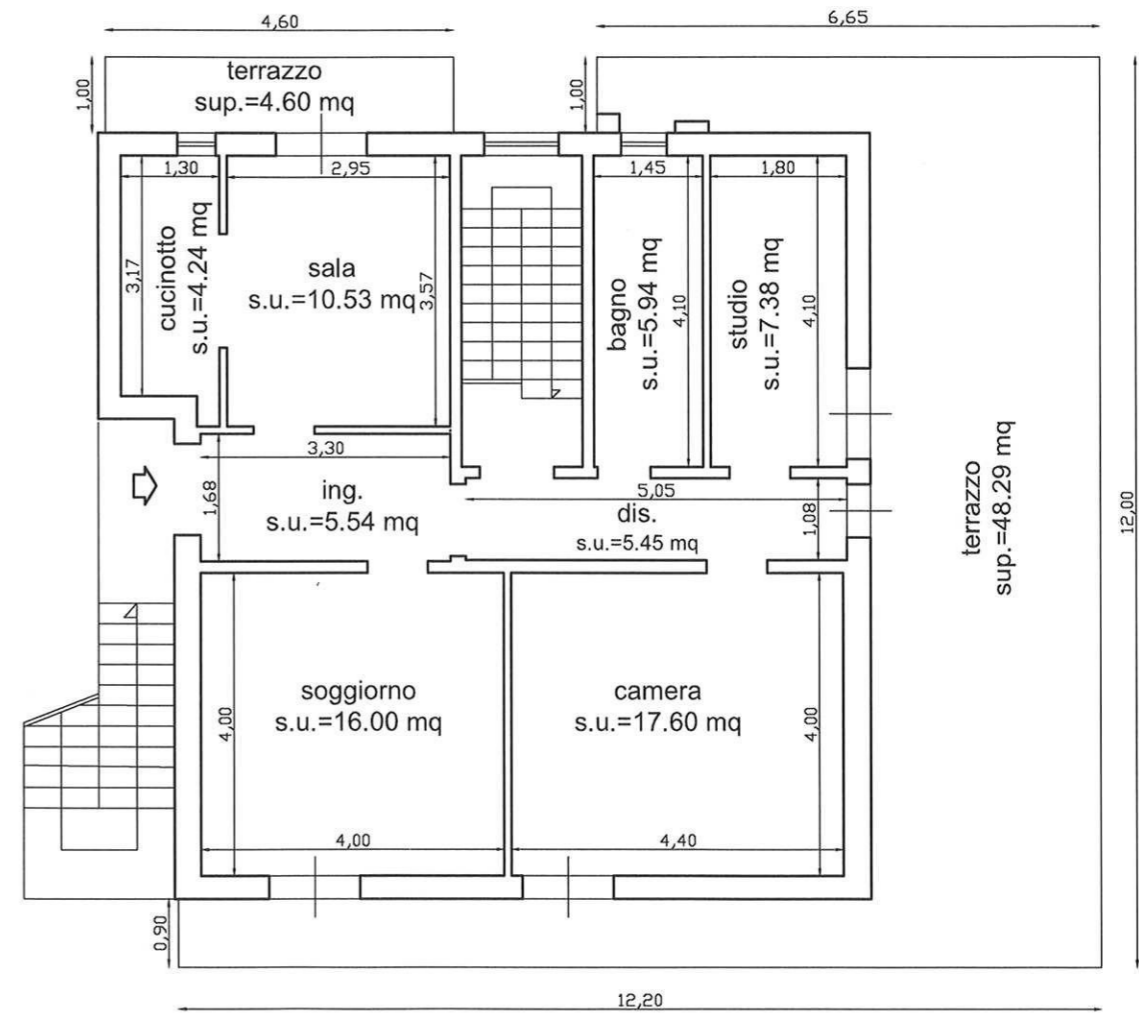
Piano Secondo h=3.00 72.68 mq
