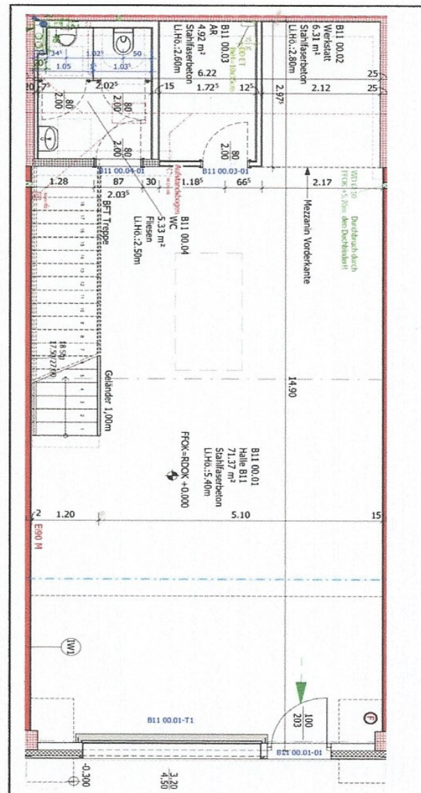
Erdgeschoss
