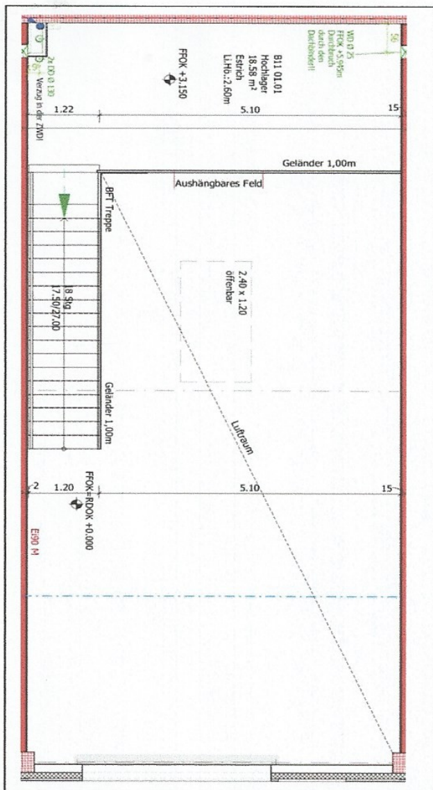
Obergeschoss
