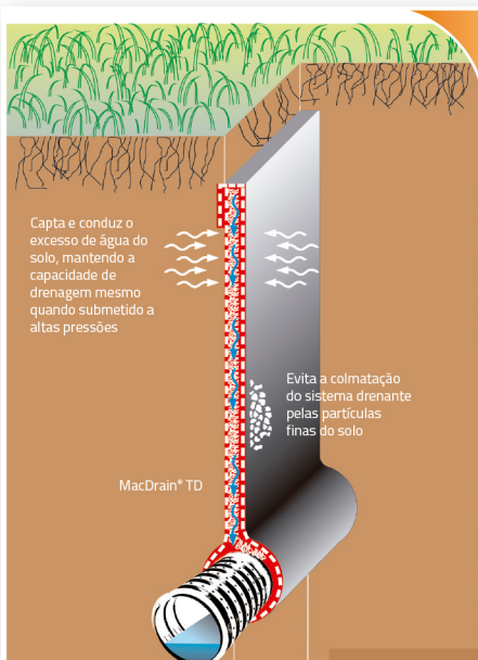
Trincheira drenante
