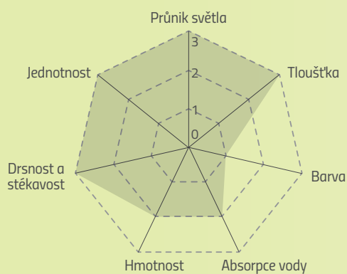
Průměrné vlastnosti georohoží
