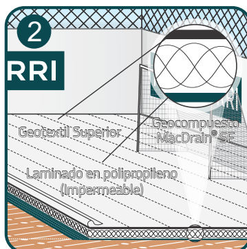
Colocación del Geocompuesto MacDrain® SF
