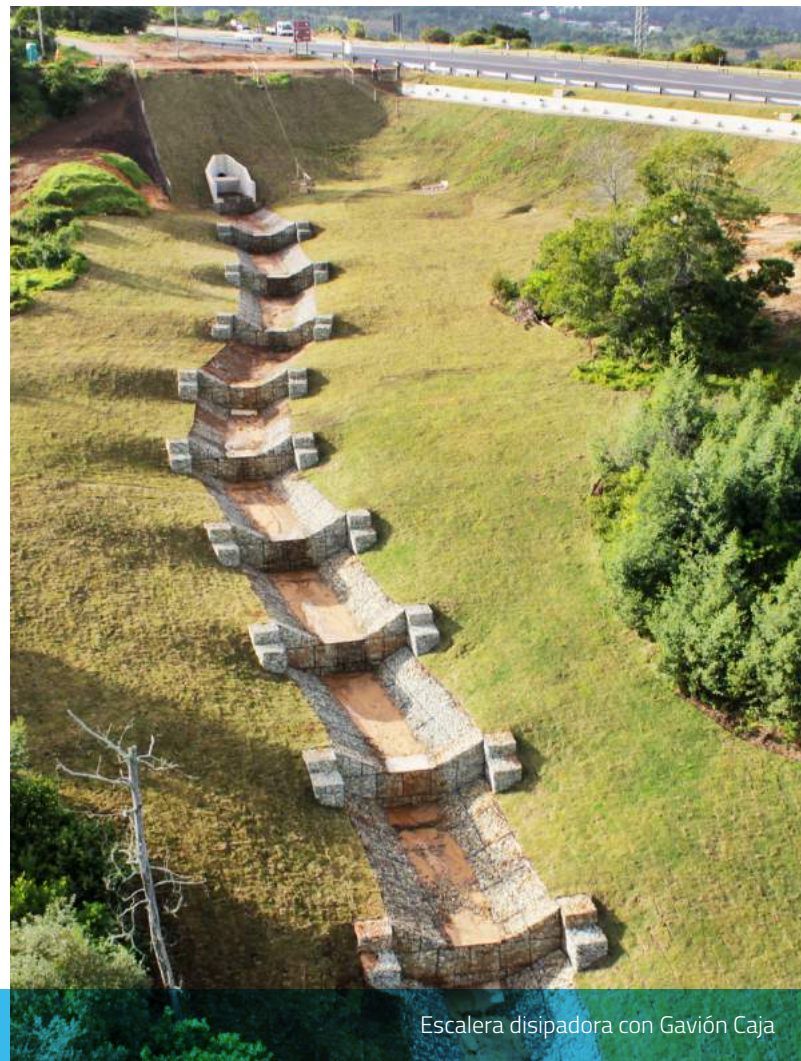
Soporte y protección de puente con Gavión Caja
