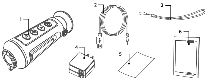
ABBILDUNG 1-2. STANDARDKOMPONENTEN
